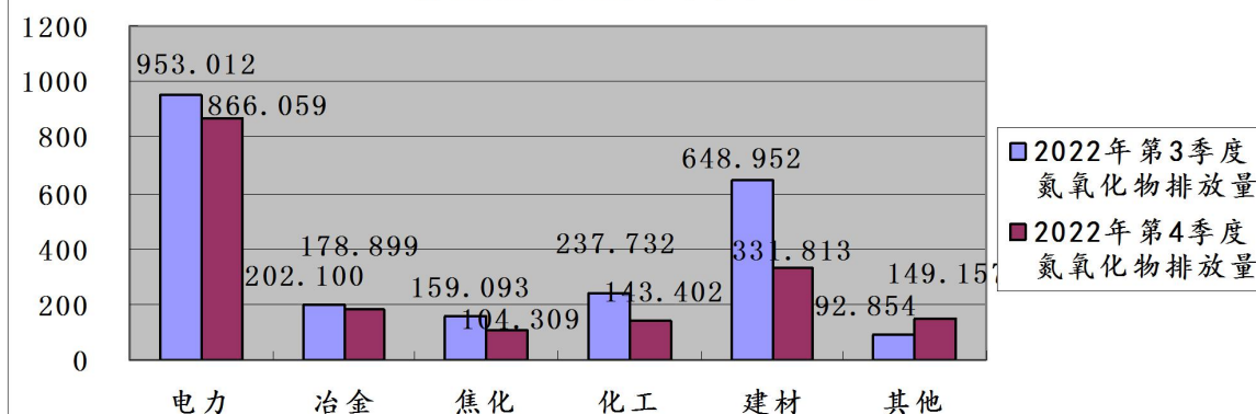
图11: 2022年第4季度晋城市监控企业废气氮氧化物 排放量环比图（单位：吨）
