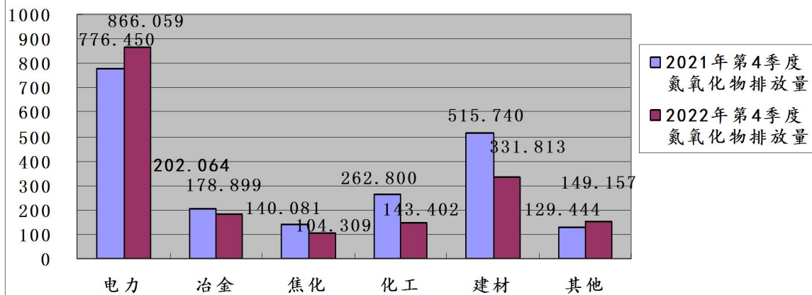
图10:2022年第4季度晋城市监控企业废气氮氧化物 排放量同比图（单位：吨）
