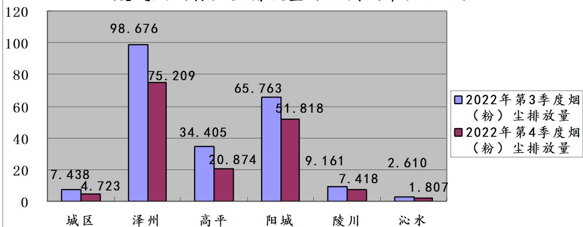
图19:2022年第4季度晋城市各县（市、区）监控企业 废气烟（粉）尘排放量环比图（单位：吨）
