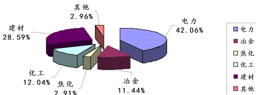
图2：2023年第2季度晋城市监控企业废气氮氧化物排放量各行业占比图
