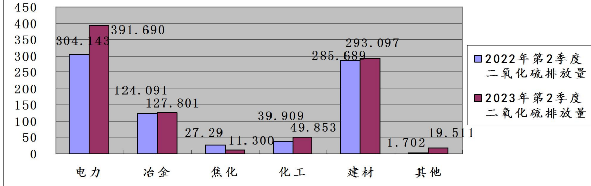
图8:2023年第2季度晋城市监控企业废气二氧化硫排放量同比图（单位：吨）
