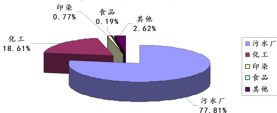
图7:2023年第2季度晋城市监控企业废水总氮排放量各行业比较图
