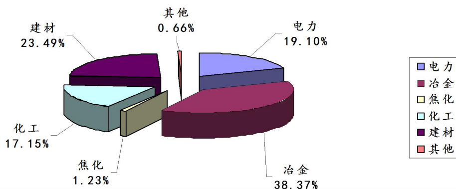
图3：2023年第2季度晋城市监控企业烟（粉）尘排放量各行业占比图
