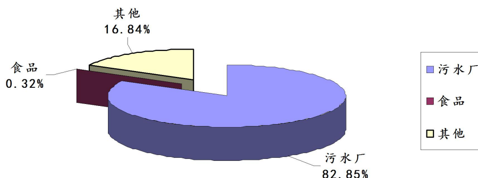
图6:2023年第3季度晋城市监控企业废水总磷排放量各行业比较图
