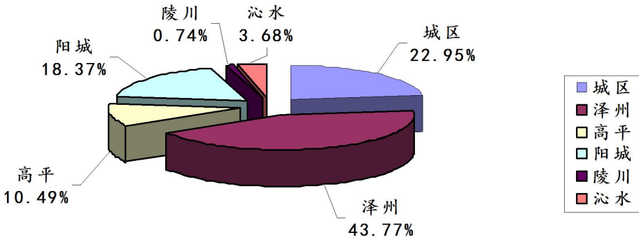
图25: 2023年第3季度晋城市各县（市、区）监控企业 废水氨氮排放量比较图
