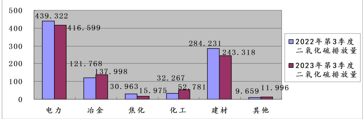
图8:2023年第3季度晋城市监控企业废气二氧化硫排放量同比图（单位：吨）
