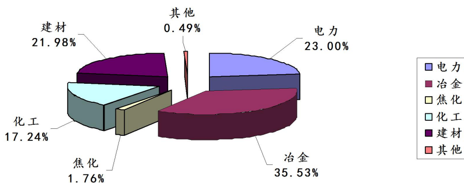
图3：2023年第3季度晋城市监控企业烟（粉）尘排放量各行业占比图
