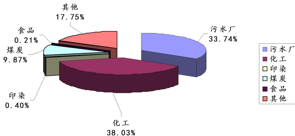
图5:2023年第3季度晋城市监控企业废水氨氮排放量各行业比较图
