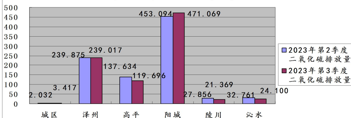
图17:2023年第3季度晋城市各县（市、区）监控企业 废气二氧化硫排放量环比图（单位：吨）
