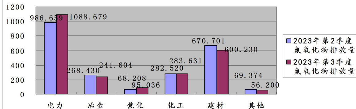
图11: 2023年第3季度晋城市监控企业废气氮氧化物 排放量环比图（单位：吨）
