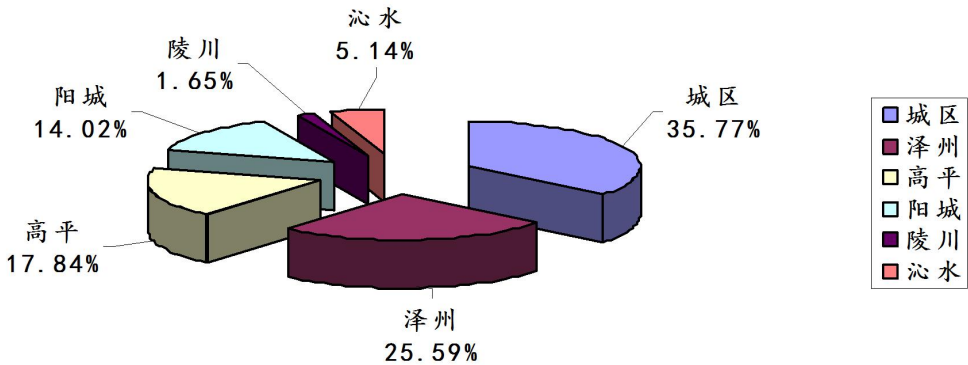
图24:2023年第3季度晋城市各县（市、区）监控企业 废水化学需氧量排放量比较图
