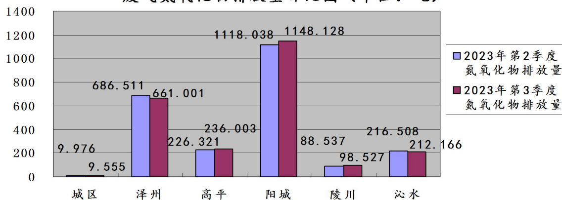
图18:2023年第3季度晋城市各县（市、区）监控企业 废气氮氧化物排放量环比图（单位：吨）
