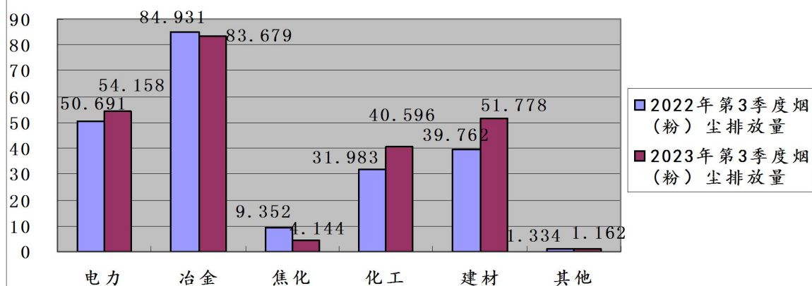
图12:2023年第3季度晋城市监控企业废气烟（粉）尘 排放量同比图（单位：吨）
