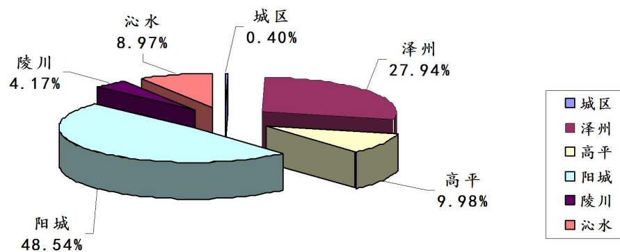
图15:2023年第3季度晋城市各县（市、区）监控企业废气 氮氧化物排放量占比图
