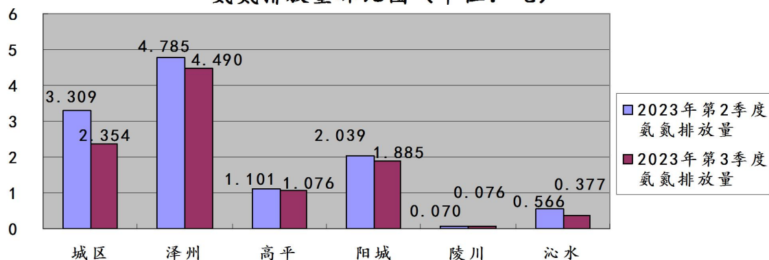
图27：2023年第3季度晋城市各县(市、区)监控企业废水 氨氮排放量环比图（单位：吨）
