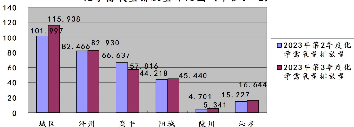
图26：2023年第3季度晋城市各县(市、区)监控企业废水 化学需氧量排放量环比图（单位：吨）
