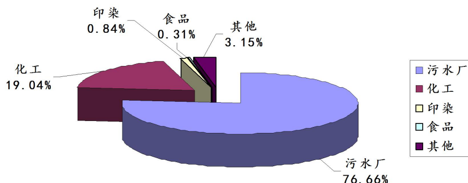
图7:2023年第3季度晋城市监控企业废水总氮排放量各行业比较图
