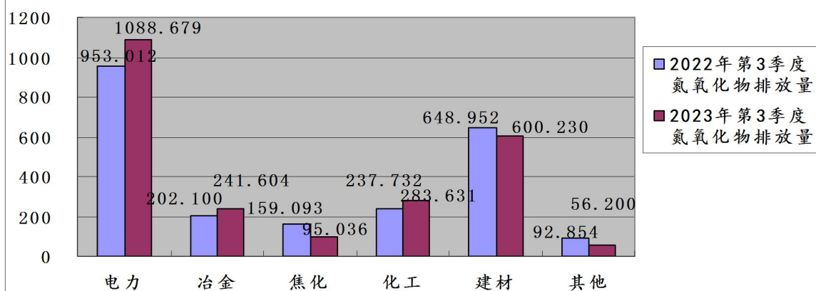
图10:2023年第3季度晋城市监控企业废气氮氧化物 排放量同比图（单位：吨）
