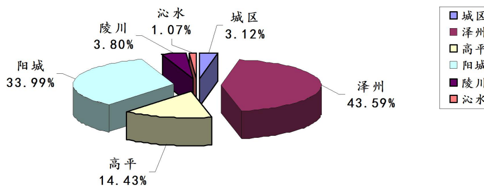
图16:2023年第3季度晋城市各县（市、区）监控企业 废气烟（粉）尘排放量占比图
