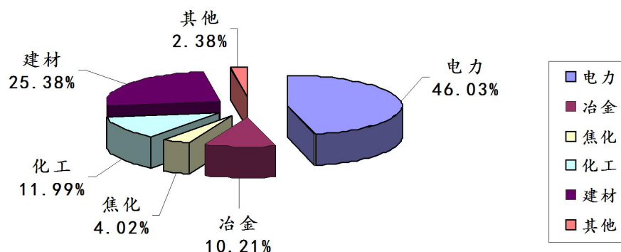
图2：2023年第3季度晋城市监控企业废气氮氧化物排放量各行业占比图
