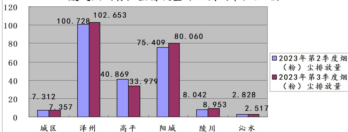
图19:2023年第3季度晋城市各县（市、区）监控企业 废气烟（粉）尘排放量环比图（单位：吨）
