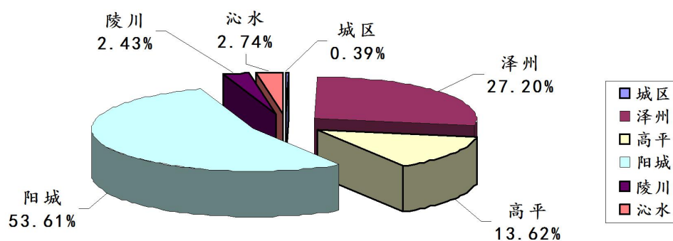
图14:2023年第3季度晋城市各县（市、区）监控企业 废气二氧化硫排放量占比图
