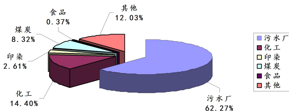
图4:2023年第3季度晋城市监控企业废水化学需氧量排放量各行业比较图
