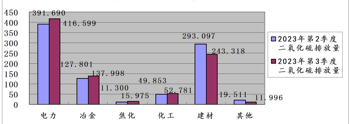
图9: 2023年第3季度晋城市监控企业废气二氧化硫排放量环比图（单位：吨）
