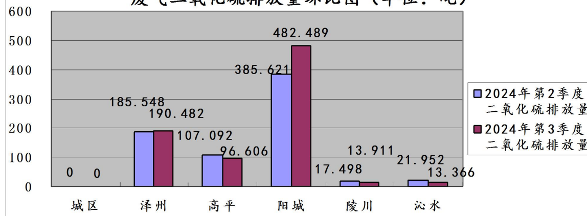
图18:2024年第3季度晋城市各县（市、区）监控企业废气二氧化硫排放量环比图（单位：吨）
