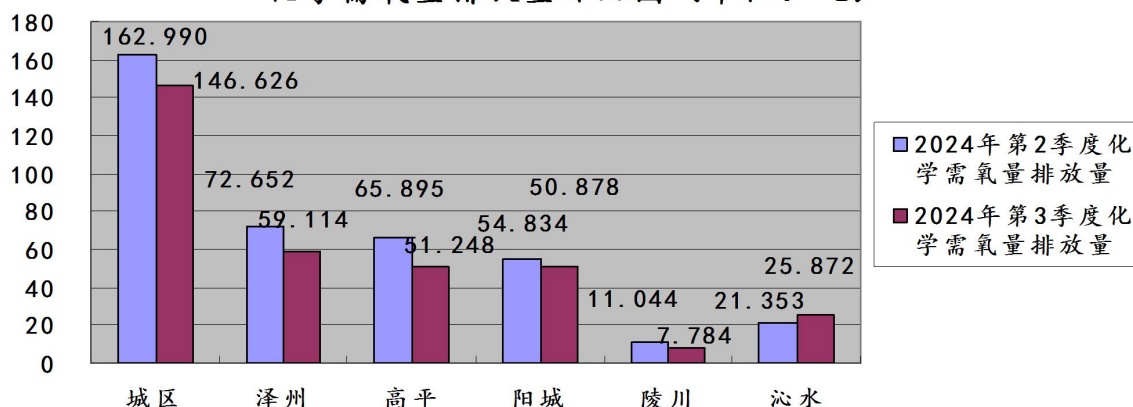
图30：2024年第3季度晋城市各县(市、区)监控企业废水 化学需氧量排放量环比图（单位：吨）
