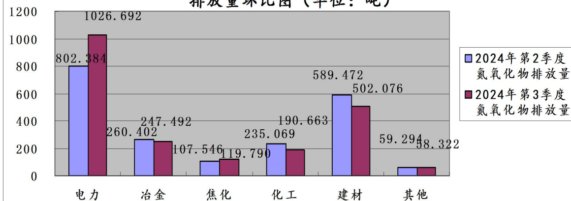
图11: 2024年第3季度晋城市监控企业废气氮氧化物 排放量环比图 (单位: 吨)
