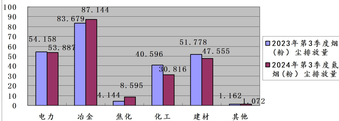
图12: 2024年第3季度晋城市监控企业废气烟(粉)尘 排放量同比图 (单位: 吨)
