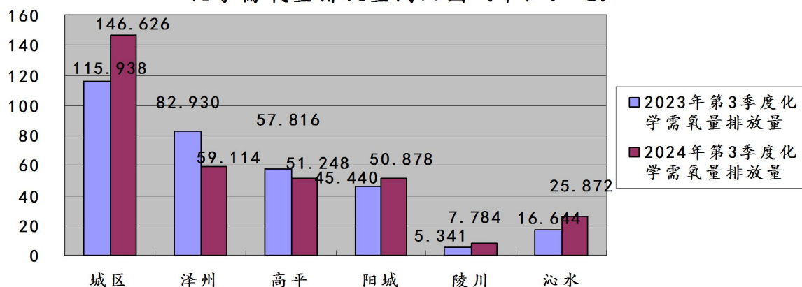
图29：2024年第3季度晋城市各县(市、区)监控企业废水 化学需氧量排放量同比图（单位：吨）
