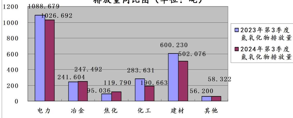
图10: 2024年第3季度晋城市监控企业废气氮氧化物 排放量同比图 (单位: 吨)
