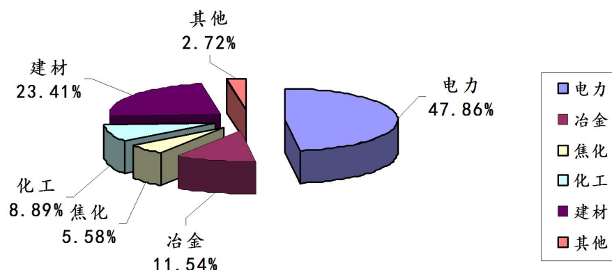
图2：2024年第3季度晋城市监控企业废气氮氧化物排放量各行业占比图
