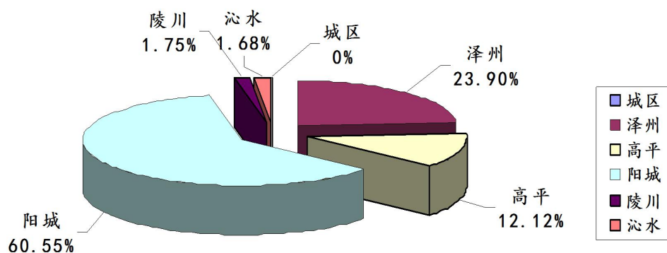
图14:2024年第3季度晋城市各县（市、区）监控企业废气二氧化硫排放量占比图
