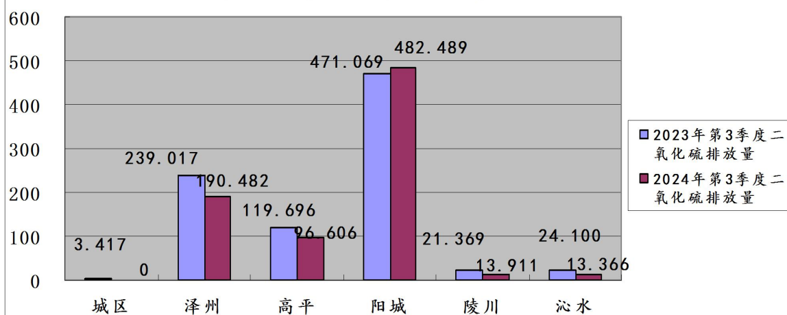
图17:2024年第3季度晋城市各县（市、区）监控企业废气二氧化硫排放量同比图（单位：吨）
