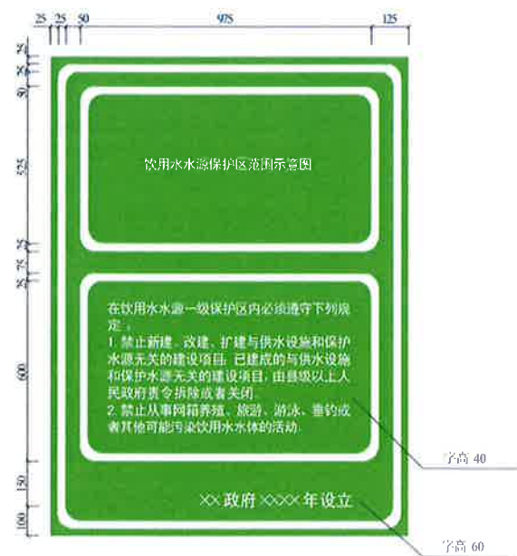
饮用水水源保护区界标背面图示及尺寸 (单位: mm)
