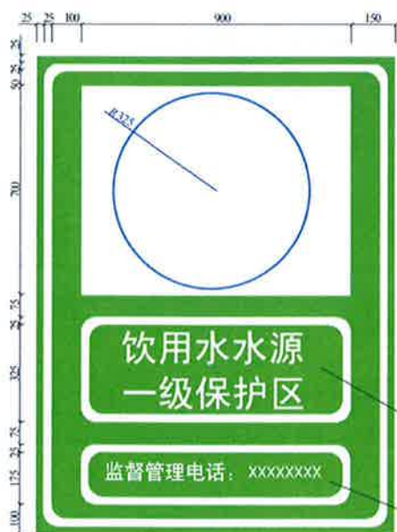
饮用水水源保护区界标正面图示及尺寸 (单位: mm)
